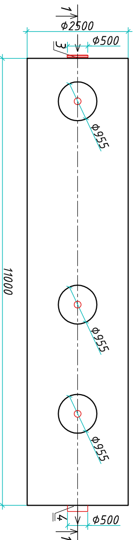
Вид сверху
