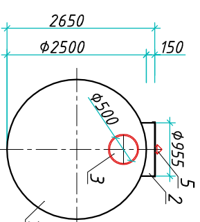
Вид А
